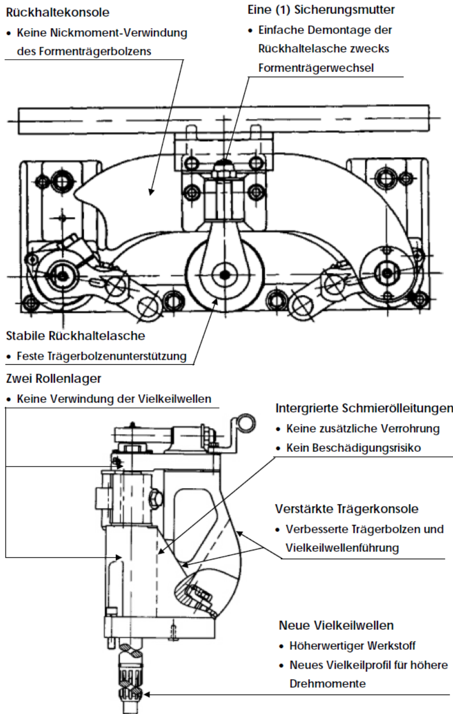
Bild 2: Vorform Trägerkonsole
