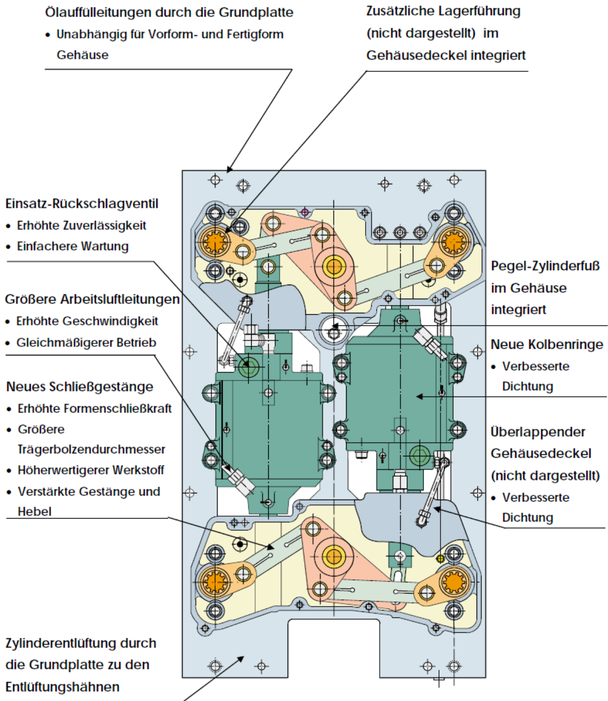
Bild 1: Formenschließmechanismus mit Schließgestänge im Ölbad
